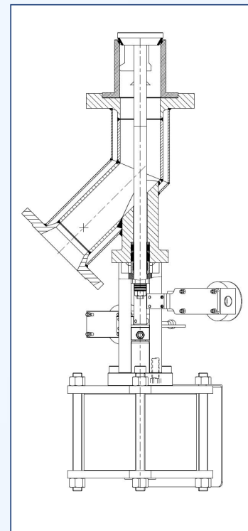
带保温夹套罐底阀
