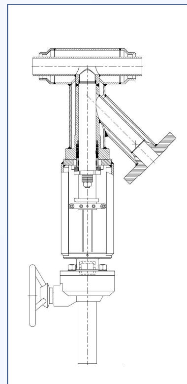
带适配管道柱塞阀 (本体密封)
