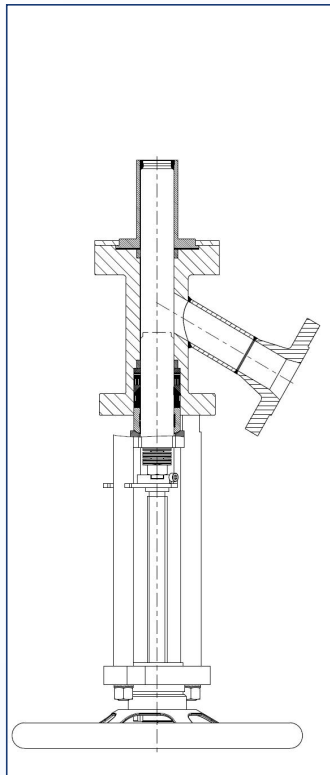
硬密封
