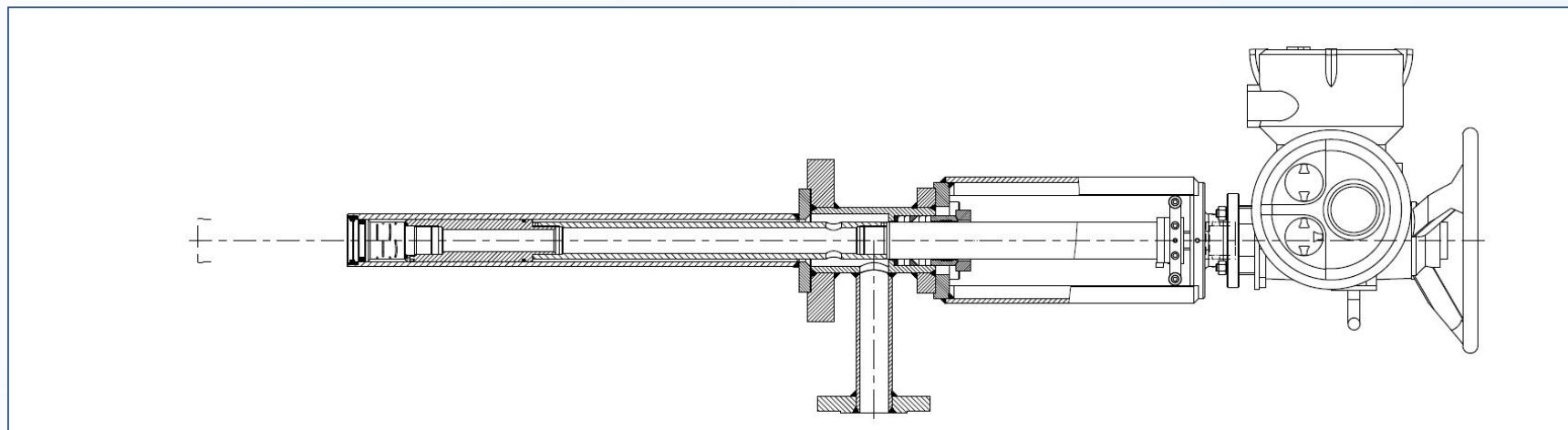
电动喷淋阀
