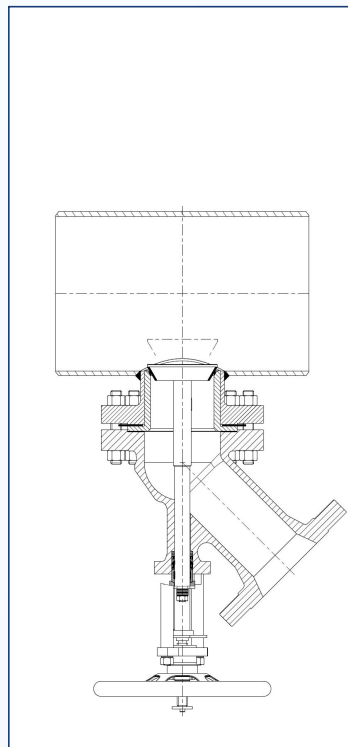
带适配管道罐底阀
