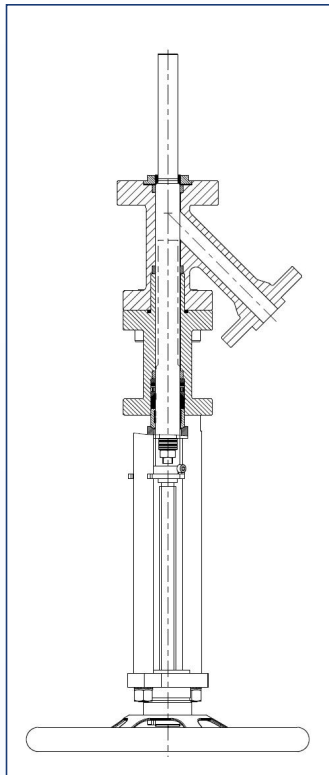
全通径硬密封
