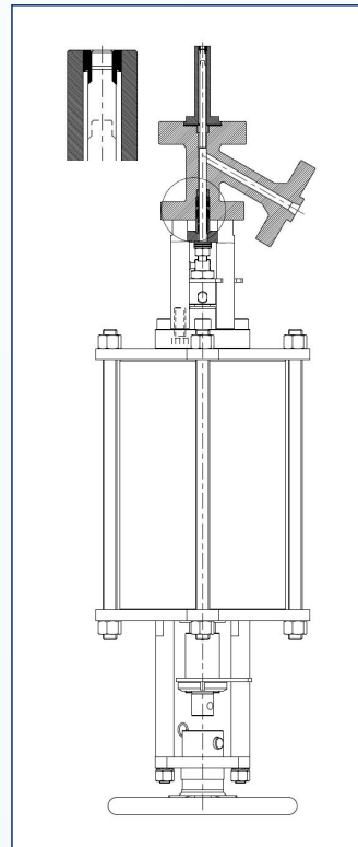
短行程硬密封
