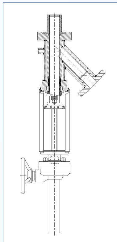
带保温夹套柱塞阀
