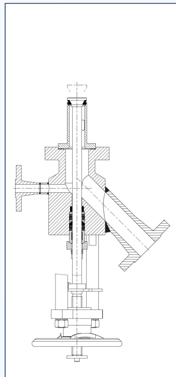
带冲洗口罐底阀
