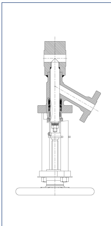
硬密封带放净环
