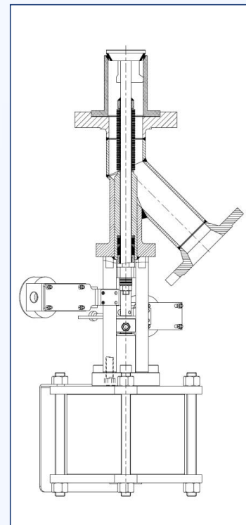
带波纹管罐底阀
