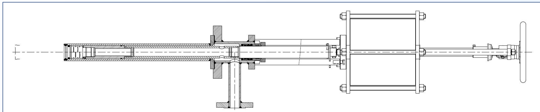
气动喷淋阀
