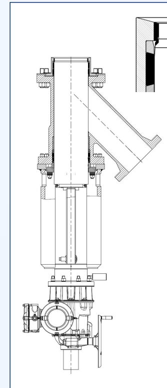
软硬双重密封密封
