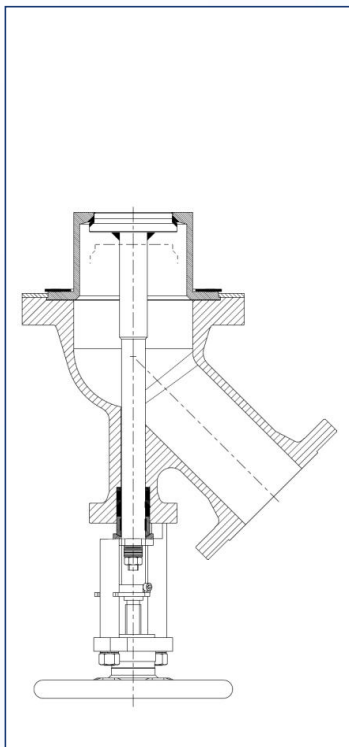
下展式罐底阀
