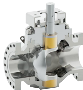
C型球阀
