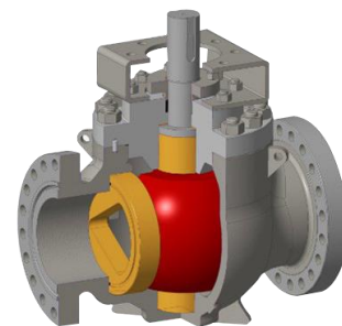
V型球阀
